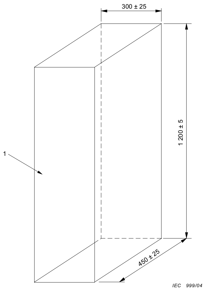
Légende 1 Face avant ouverte (tous les autres côtés sont fermés)
